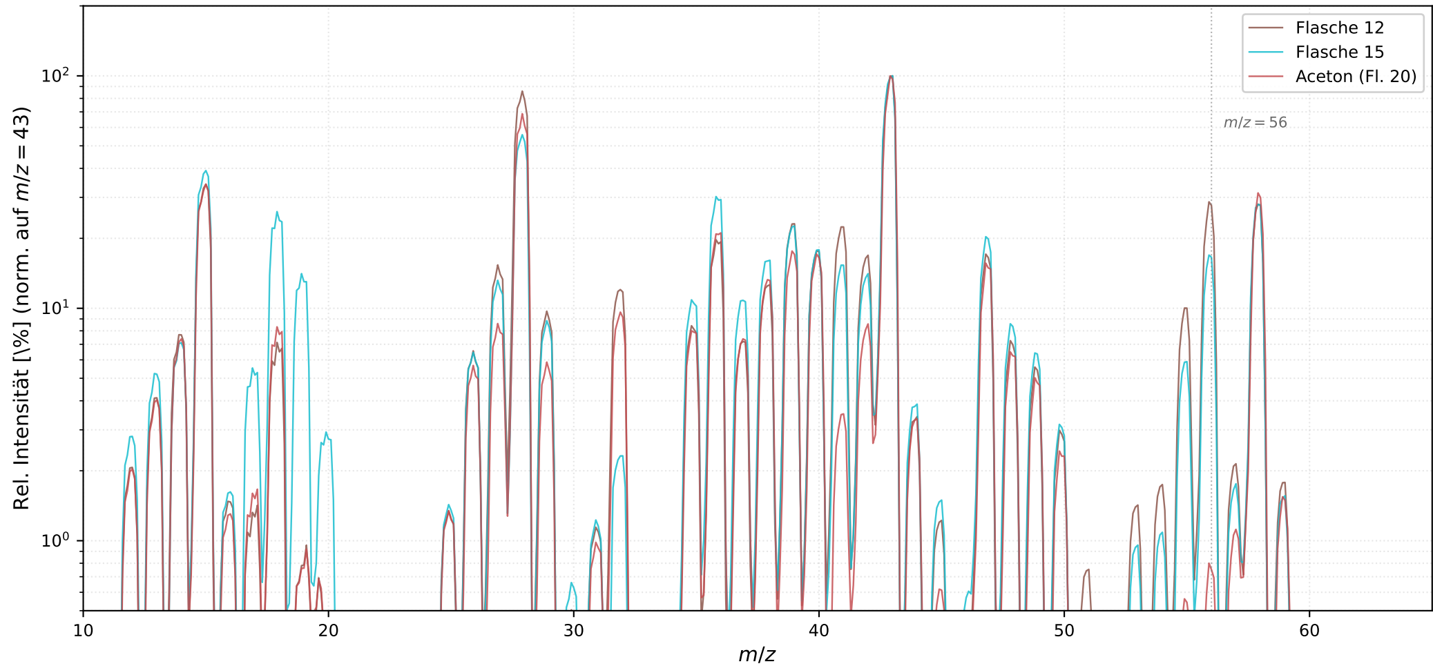
Vergleich Flasche 12, 15 und Aceton (BG-korrigiert)
